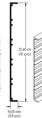
ANGLE BISEAUTÉ
